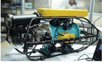
ROV MIKROS
